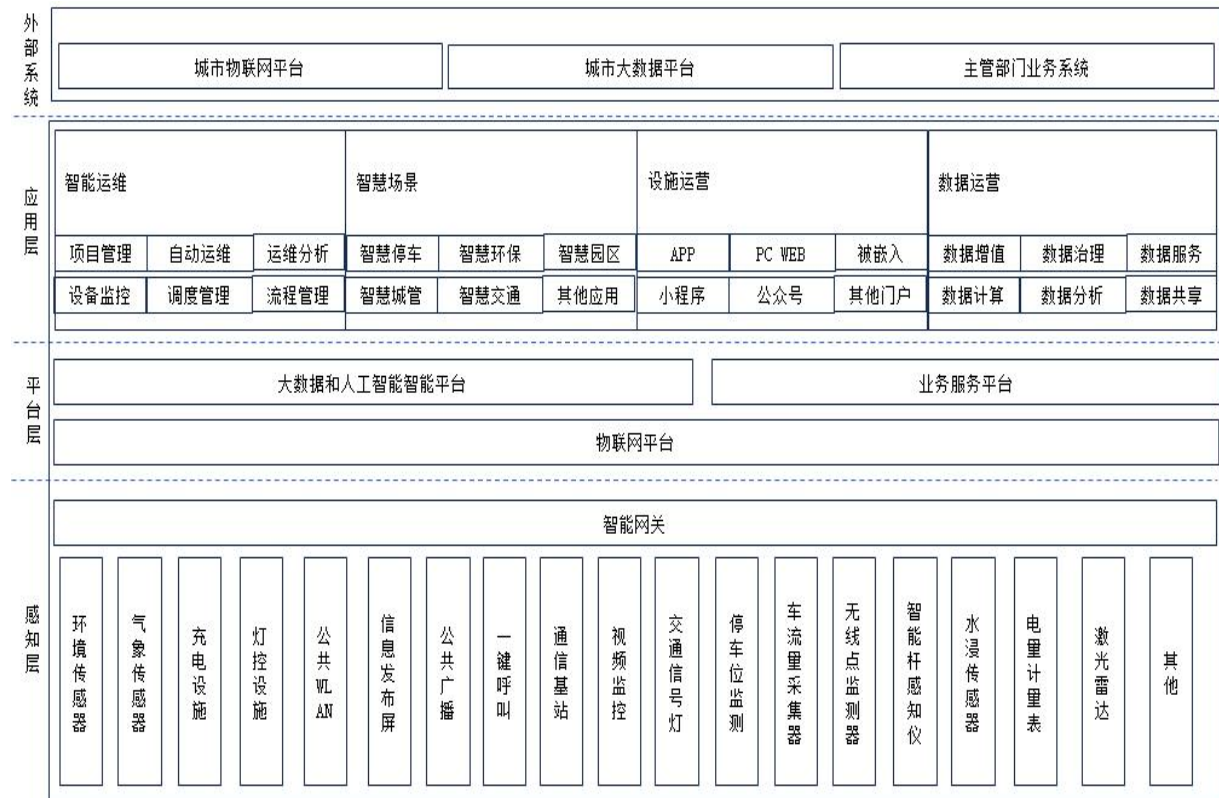
图 F.2 管理平台架构图
